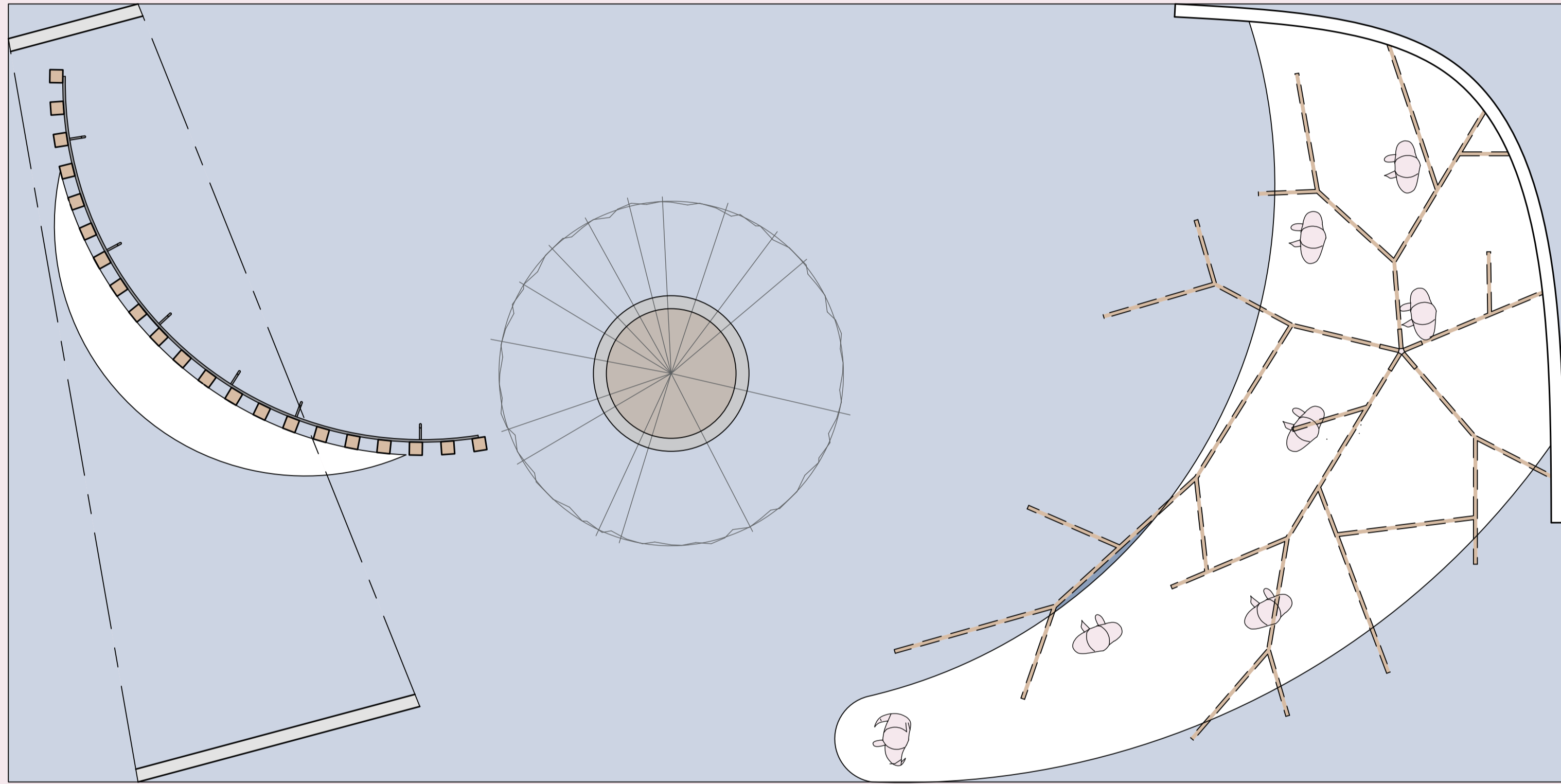
平面図 S=1/30
