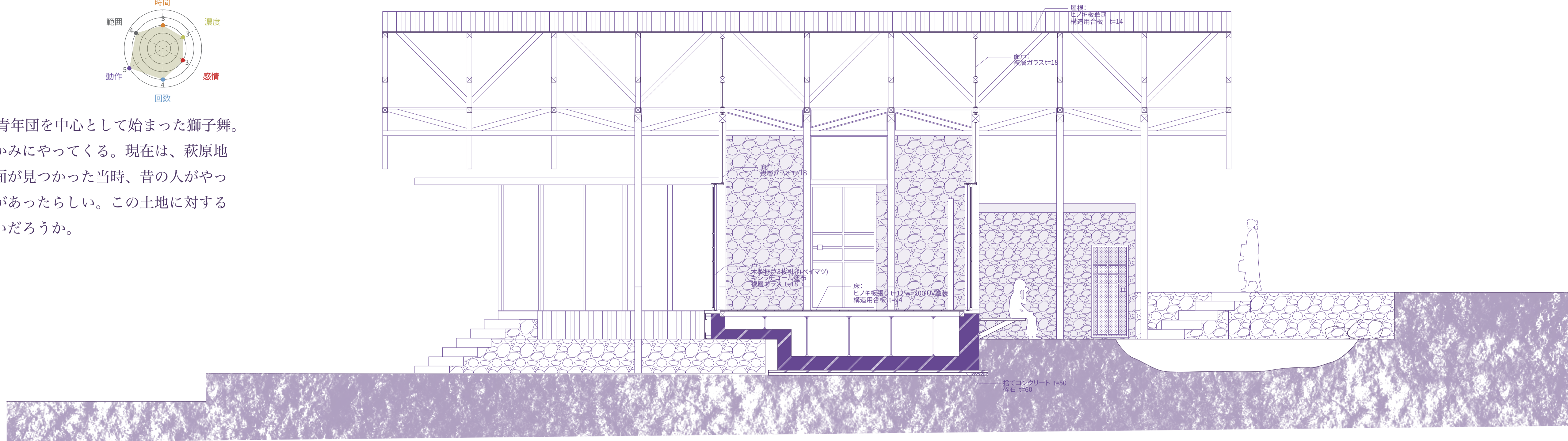
RITO-ENTEI AA' 断面図 S=1:100
