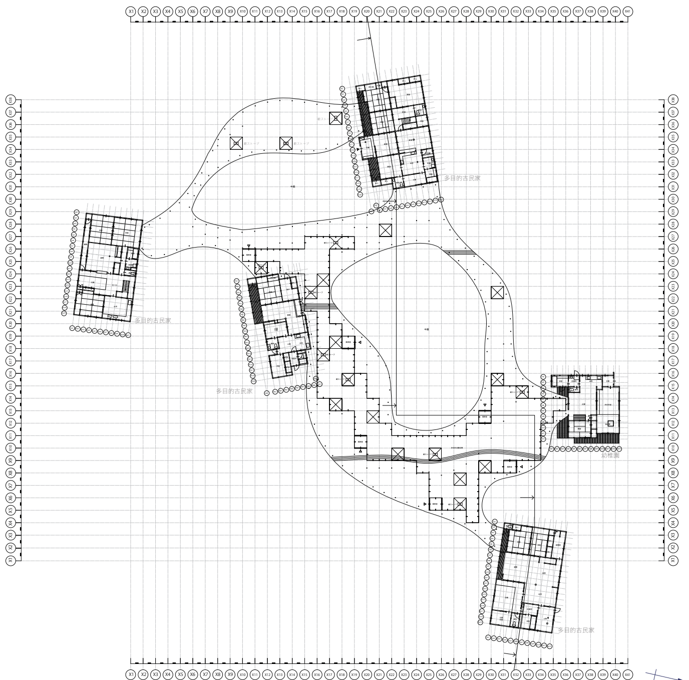
クラスター4 平面図 S=1:200
