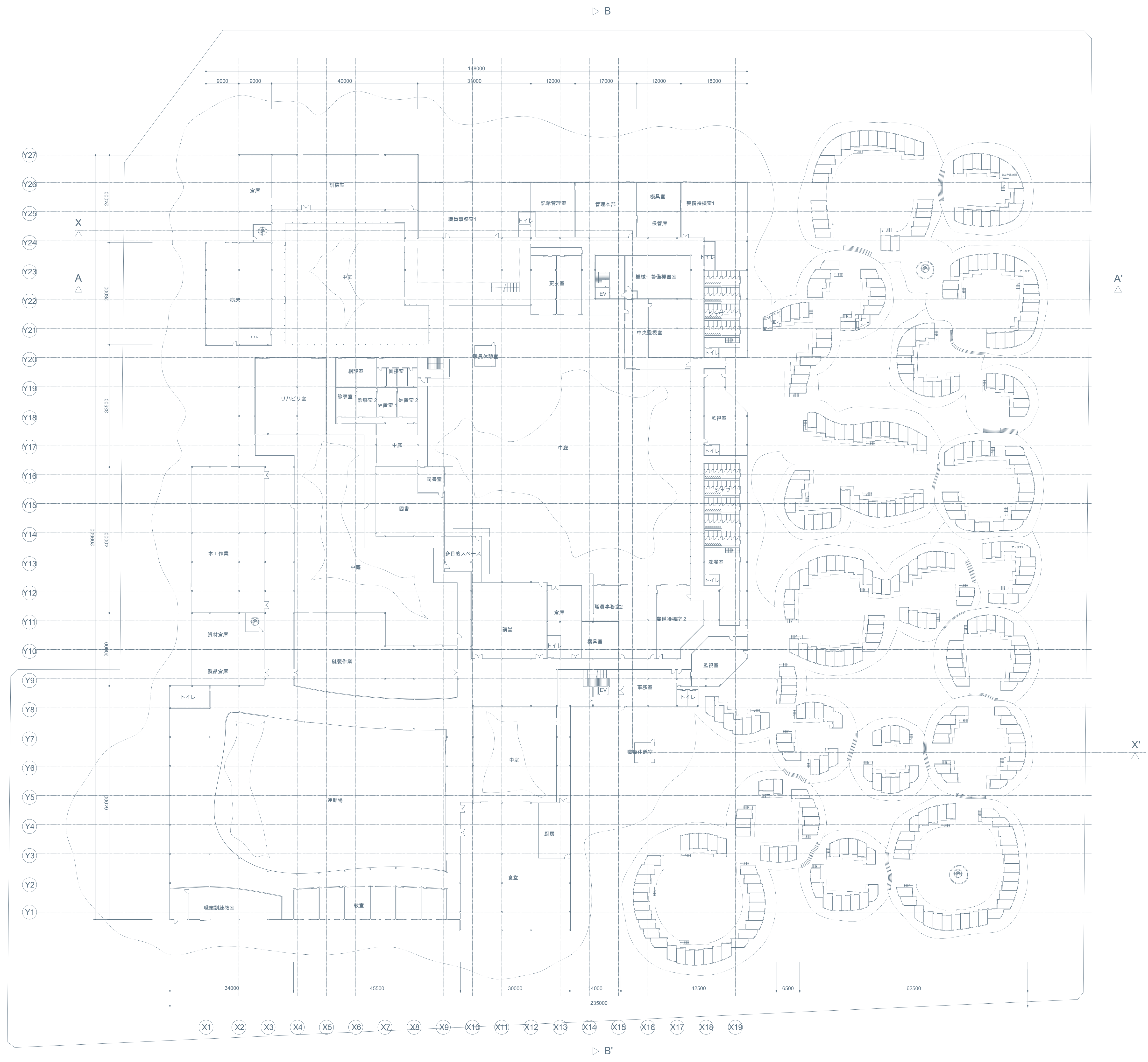
3F 平面図
