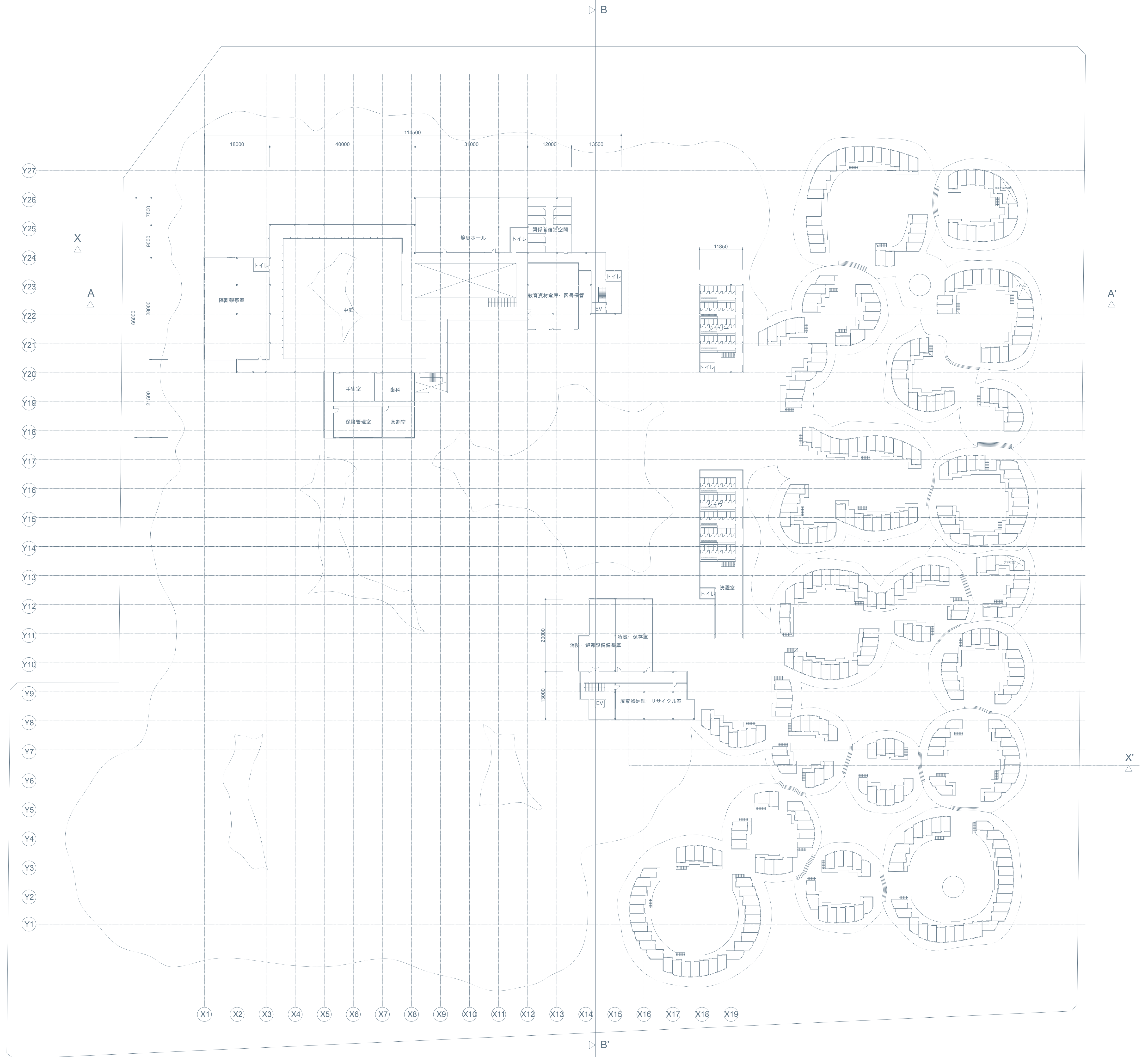
4F 平面图
